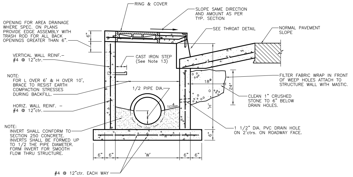
SECTION D-D
