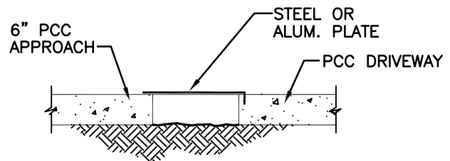
alt. SECTION A-A
