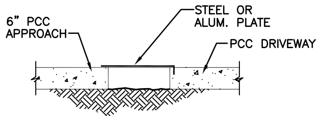
alt. SECTION A-A
