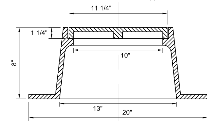
FRAME & LID
