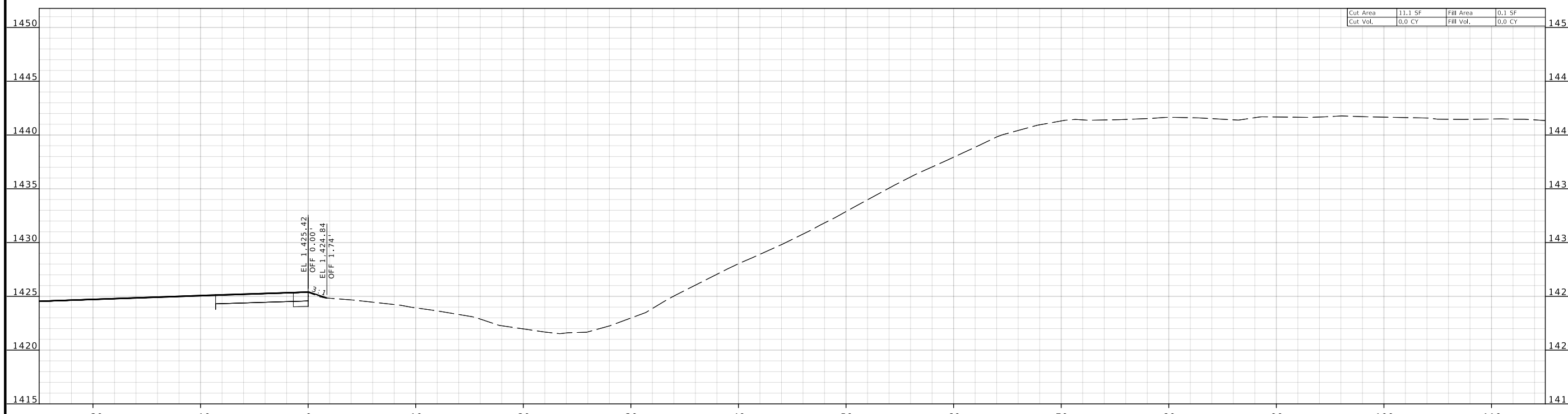
NE RADIUS STA 0+00.00
