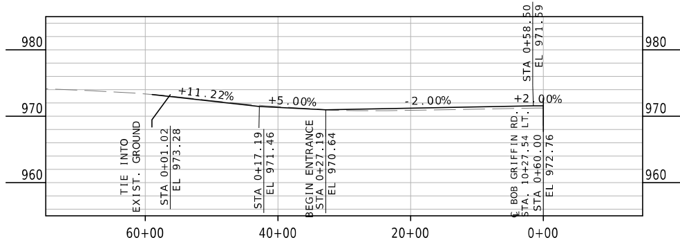
S. BOB GRIFFIN RD. - STA. 10+27.54 LT.
