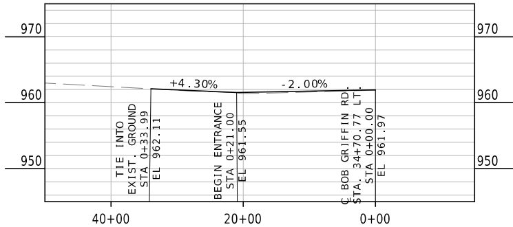
S. BOB GRIFFIN RD. - STA. 34+70.77 LT.
