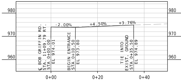
S. BOB GRIFFIN RD. - STA. 11+09.79 RT.
