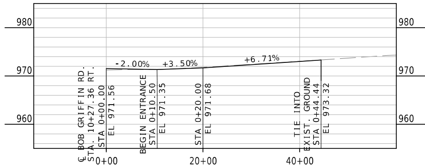
S. BOB GRIFFIN RD. - STA. 10+27.36 RT.
